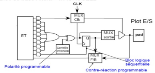
Bloc de base Altera = MACROCELL
