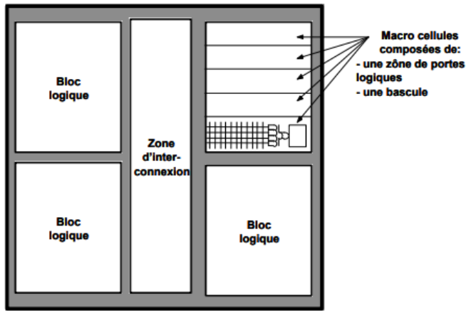
Bloc de base Altera = MACROCELL
