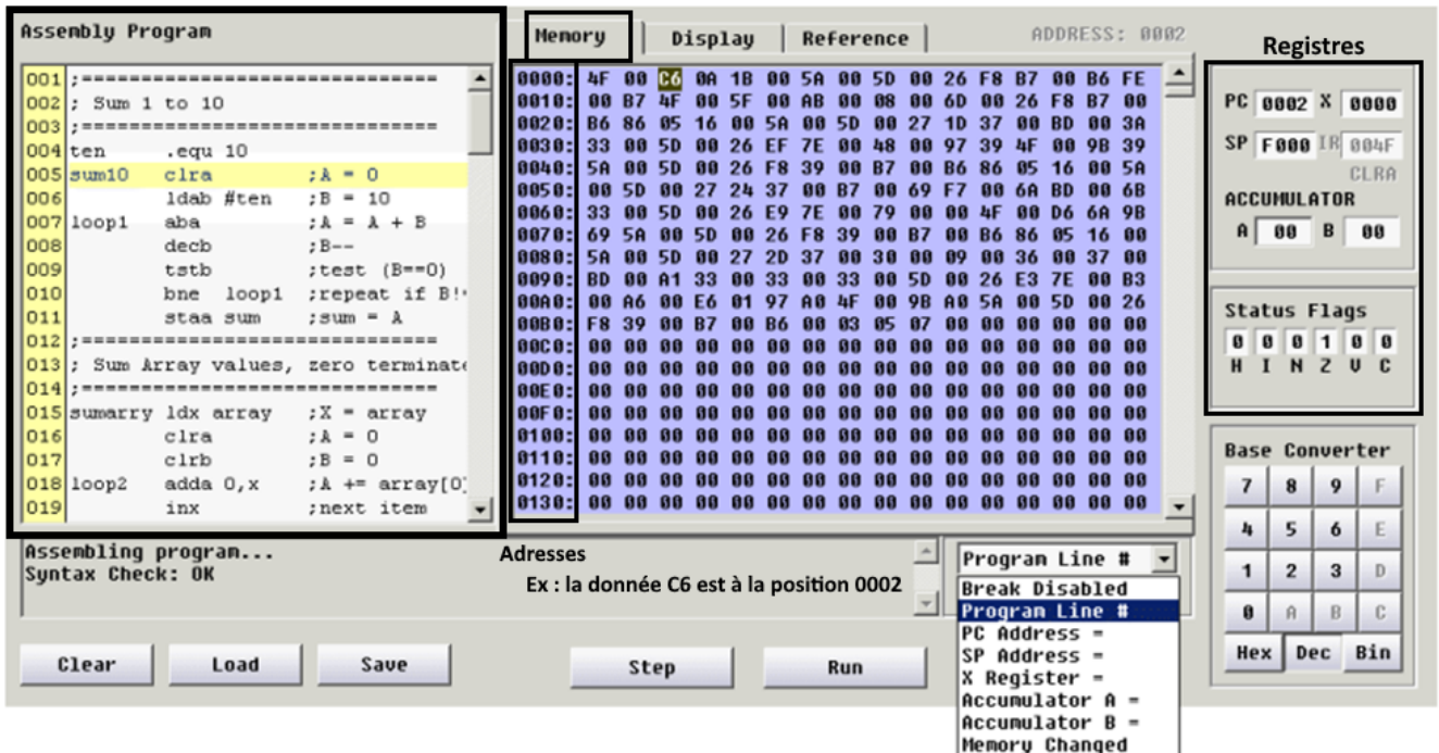
Code source en assembleur 6800/11
